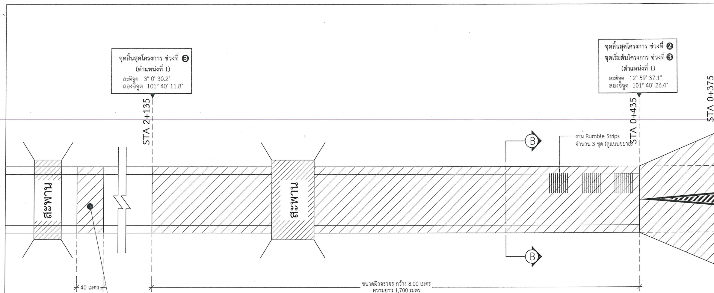
แปลนถนนแอสฟัลท์ติกคอนกรีต (ต่อ)
